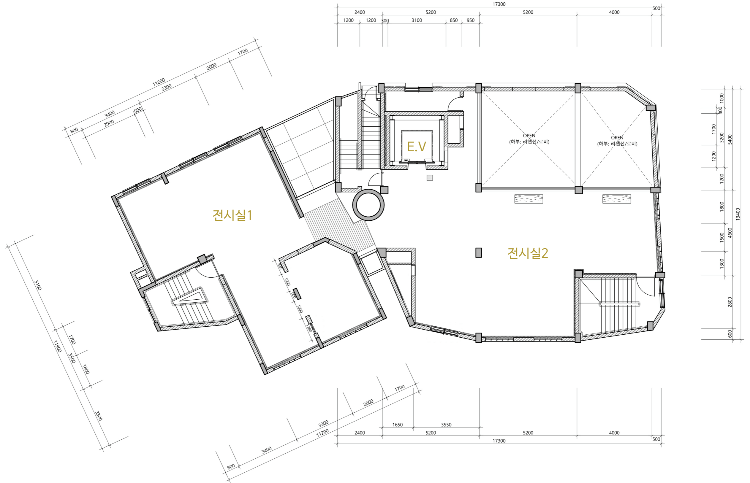
〈산지천갤러리 2층 평면도〉
